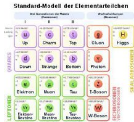
Abb. J.2.E Elementarteilchen [Wikipedia].
