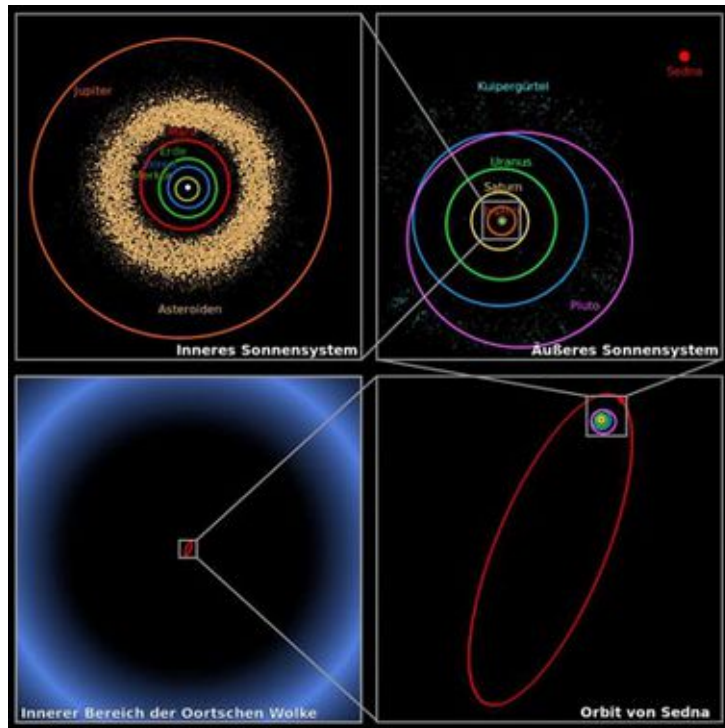
Abb. J.2.O Oortsche Wolke [Wikipedia].
