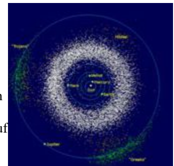
Abb. J.2.A Asteroidengürtel. [Wikipedia].
